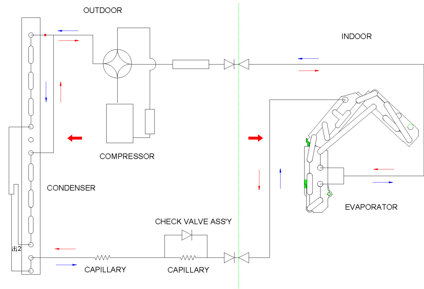
4-1. Схема циркуляции хладагента:
