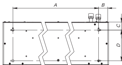
Вид сзади для ZVV-IWI0 и ZVV-2W25
