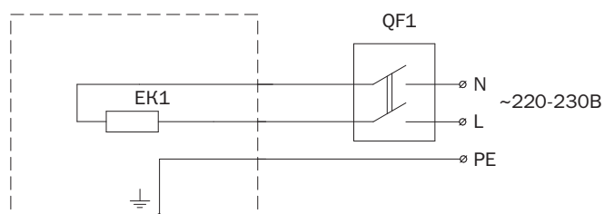
Схема электрическая IR-0.6SN3, IR-0.8SN3, IR-1.0SN3, IR-1.4SN3, IR-1.5SN3
