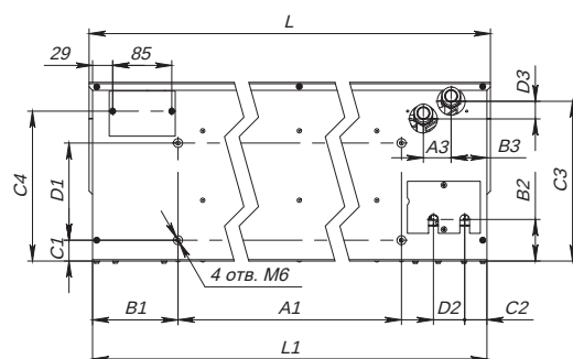
Вид снизу для ZVV-IWI0 и ZVV-2W25
