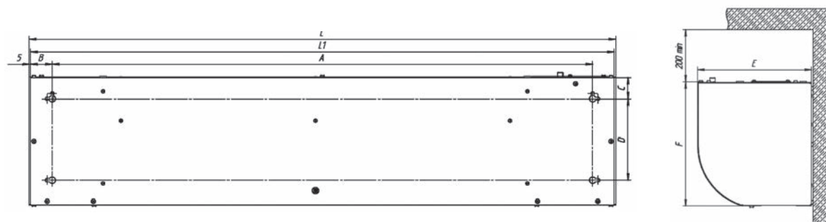
Вид сзади для ZVV-IE6T, ZVV-9T, ZVV-I.0E9T, ZVV-2EI2T, ZVV-2EI8T и ZVV-2E24T
