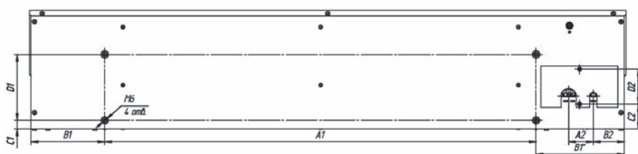
Вид снизу для ZVV-IE6T, ZVV-9T, ZVV-I.0E9T, ZVV-2EI2T, ZVV-2EI8T и ZVV-2E24T
