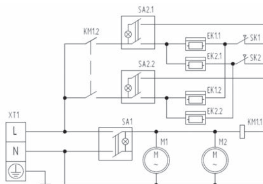
Схема электрическая ZVV-0.8E5M, ZVV-0.8E5MG
