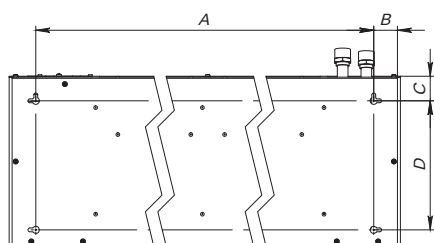
Вид сзади для ZVV-IWI5, ZVV-I.5W25 и ZVV-2W40
