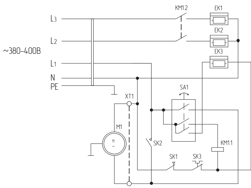
Схема электрическая ZTV-6C, ZTV-9C
