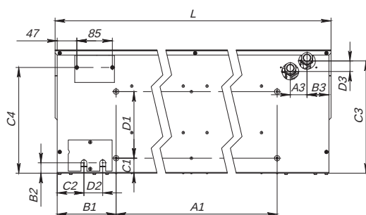
Вид снизу для ZVV-IWI5, ZVV-I.5W25 и ZVV-2W40
