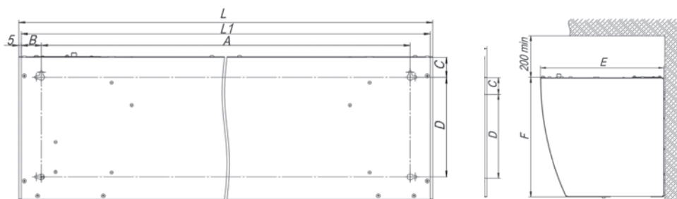
Вид сзади для ZVV-1.5E18HP
