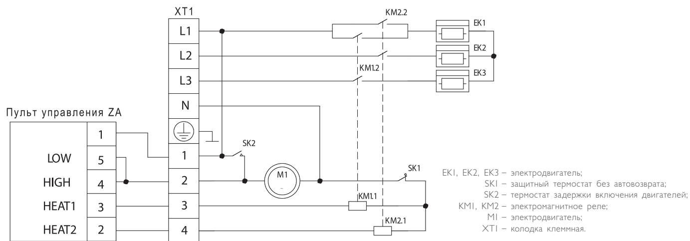
Схема электрическая ZVV-2EI8T, ZVV-2E24T
