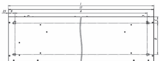
Вид сзади для ZVV-2E24HP и 2E36HP
