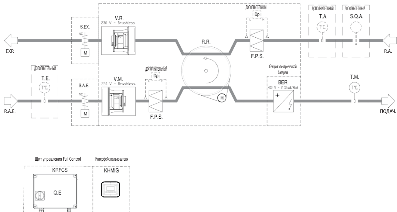
Блок рекуперации UTNRE-HE
