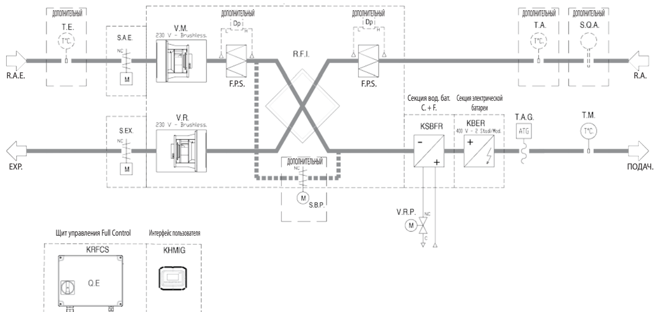
Блок рекуперации UTNRE-A/P
