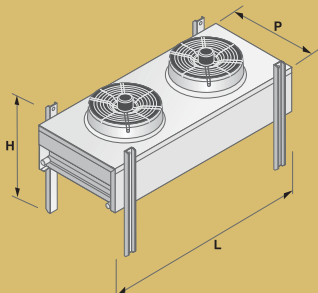
Горизонтальная установка
